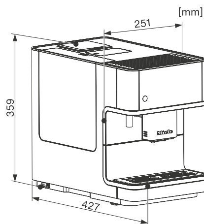
Dimensiones CM 6000
