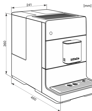
Dimensiones CM 5000
