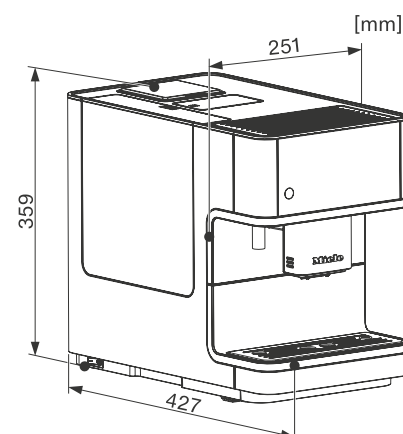
Dimensiones CM 6000
