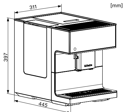
Dimensiones CM 7000
