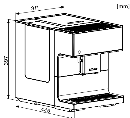
Dimensiones CM 7750
