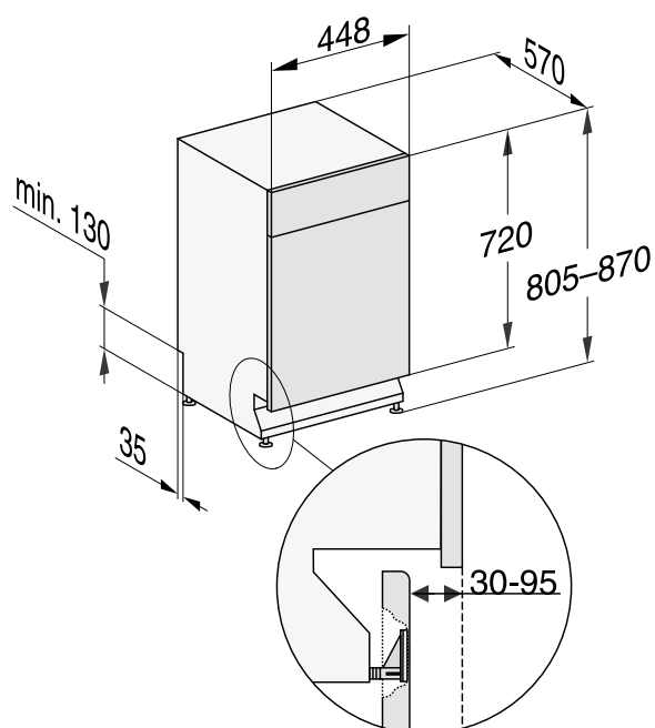
Lavavajillas empotrable bajo encimera de 45 cm
