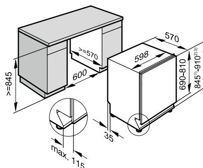
Croquis de empotramiento
