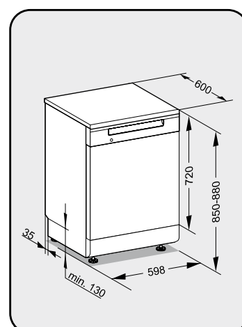
Croquis de empotramiento
