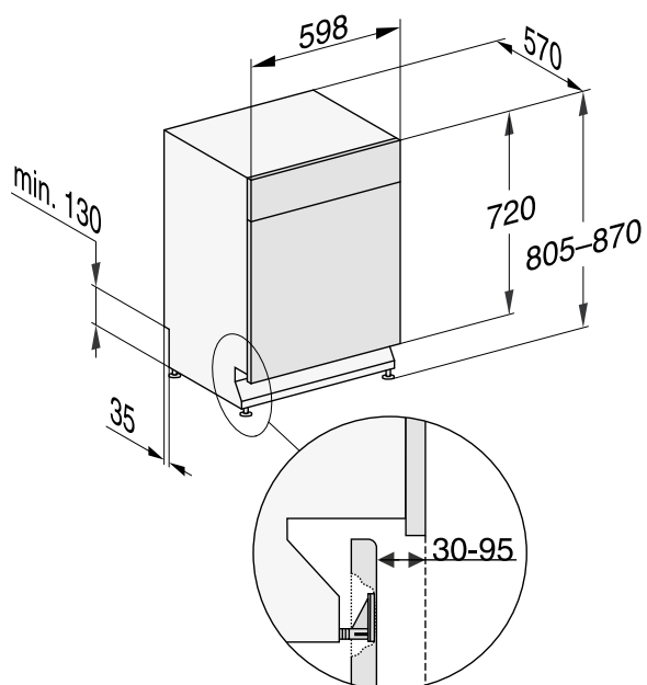
Lavavajillas empotrable bajo encimera de 60 cm
