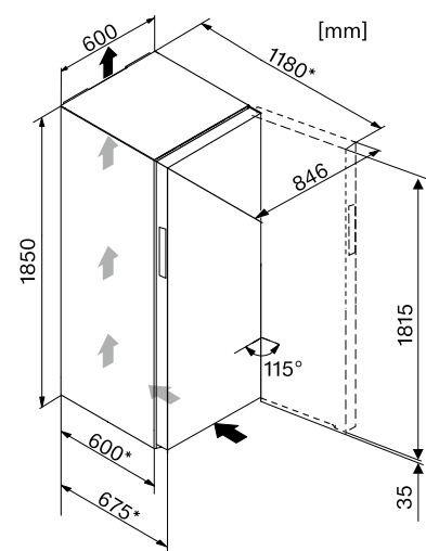
Croquis de empotramiento
