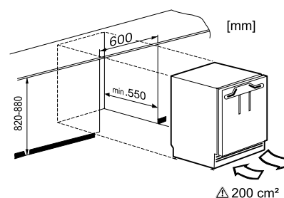
Croquis de empotramiento
