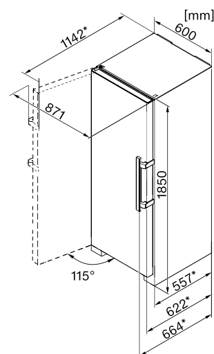
Croquis de empotramiento
