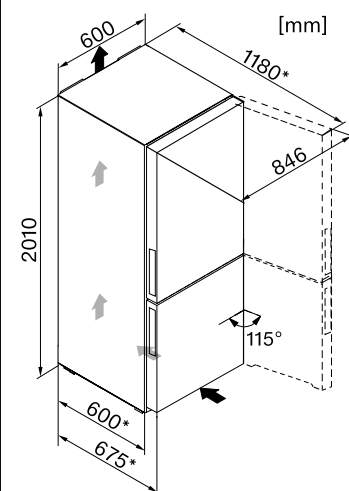
Croquis de empotramiento
