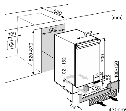
Croquis de empotramiento
