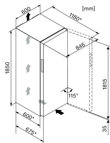
Croquis de empotramiento
