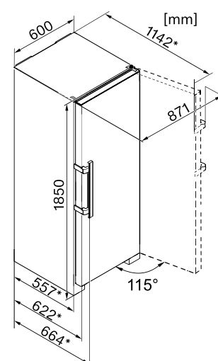
Croquis de empotramiento
