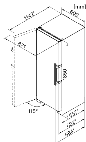
Croquis de empotramiento
