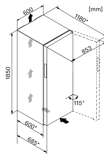
Croquis de empotramiento
