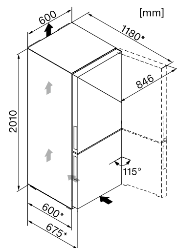
Croquis de empotramiento
