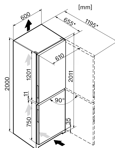
Croquis de empotramiento
