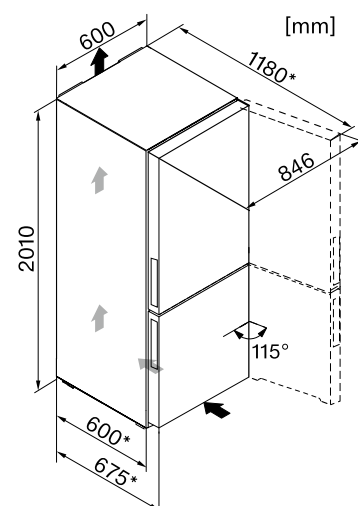
Croquis de empotramiento
