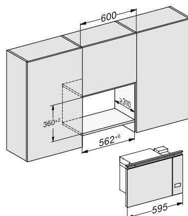
Instalación en armario superior
