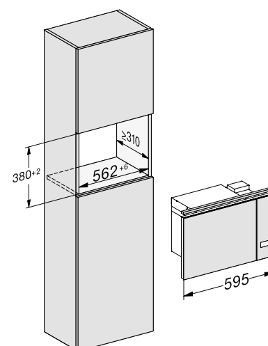
Instalación en armario alto
