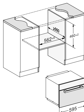
Instalación en armario superior
