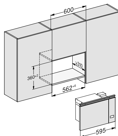
Instalación en armario superior
