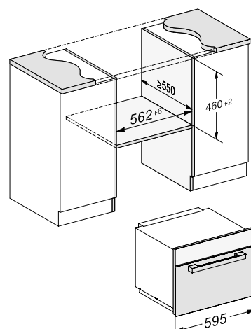
Instalación en armario superior
