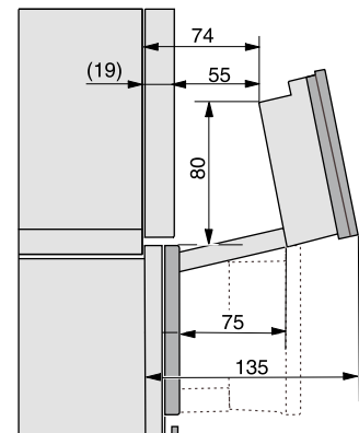
Detalle apertura panel elevable
