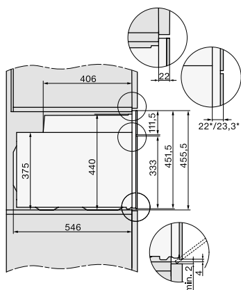
Vista lateral horno de 45 cm
