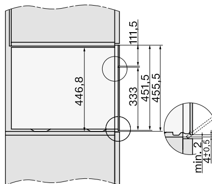
Vista lateral del hueco de 45 cm DGC XL
