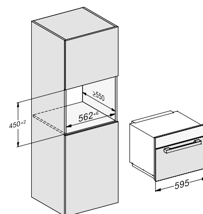
Instalación en armario alto
