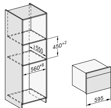
Instalación en armario superior
