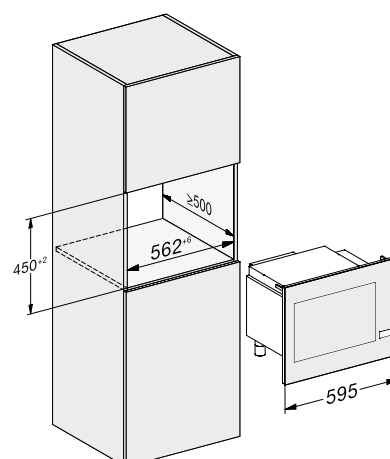
Instalación en armario alto
