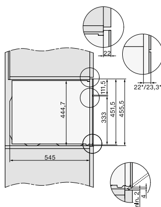
Vista lateral horno combinado con microondas de 45 cm
