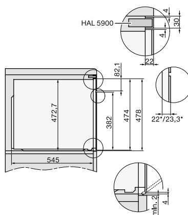
Vista lateral horno de 90 cm
