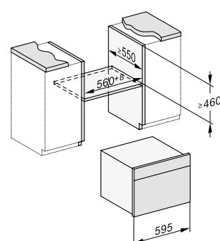
Instalación en armario alto
