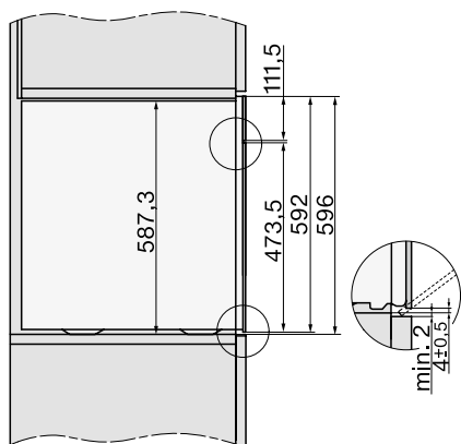
Vista lateral del hueco de 60 cm DGC XXL
