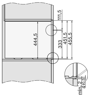
Vista lateral del hueco de 45 cm DG/DGM
