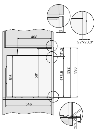
Vista lateral horno de 60 cm
