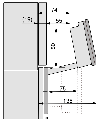
Detalle apertura panel elevable
