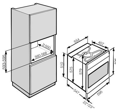
Croquis general hornos empotramiento
